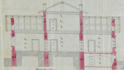
Průřez 1. patra
